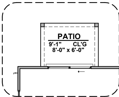
6068 Sliding Glass Door
