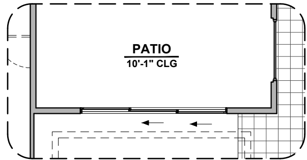
Stacking Door ILO Standard Door
