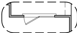
Center Hinge Door ILO Sliding Glass Door
