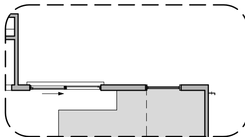
Sliding Glass Door ILO STD. Door
